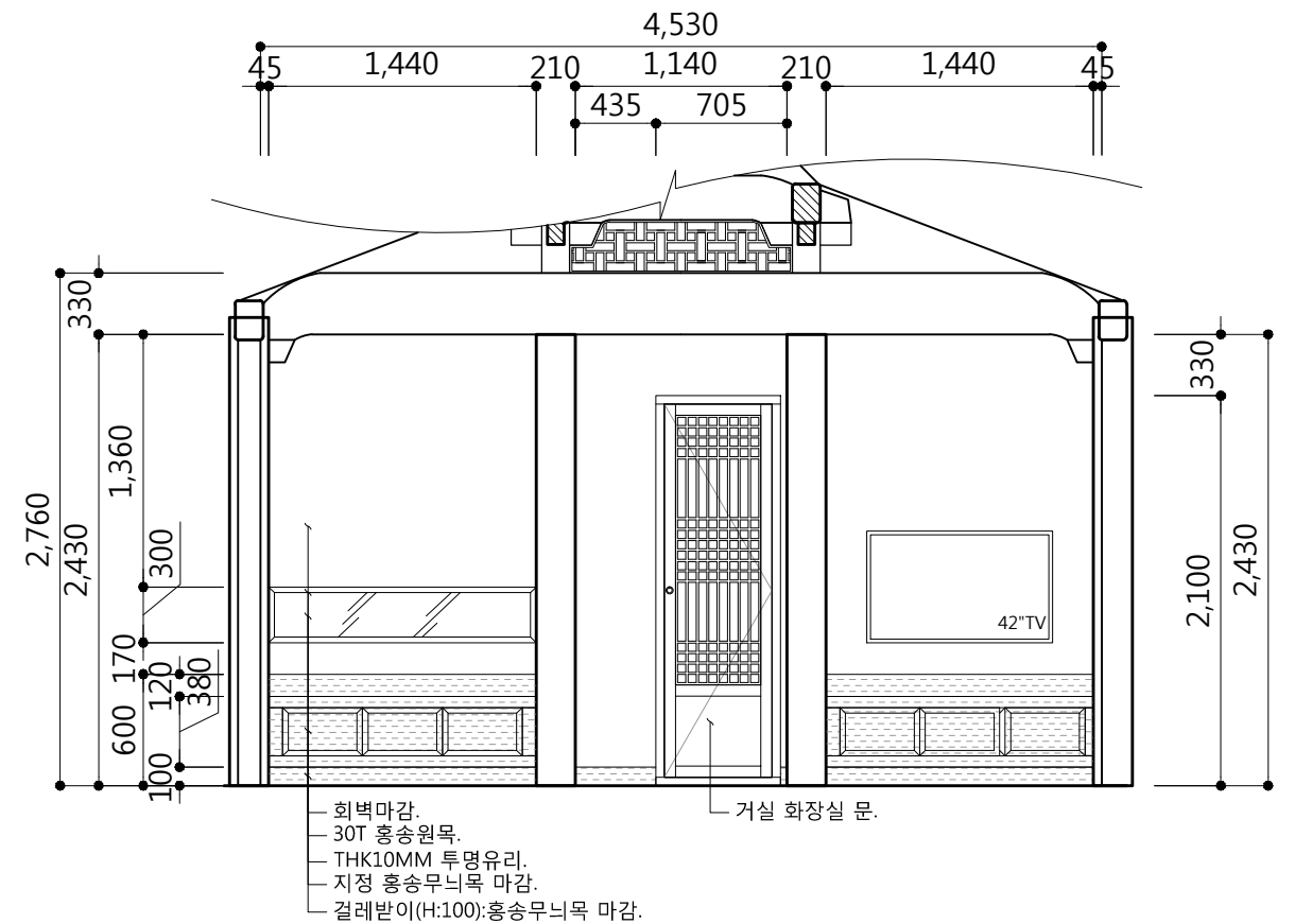
2 전통형 거실 ELEVATION B
