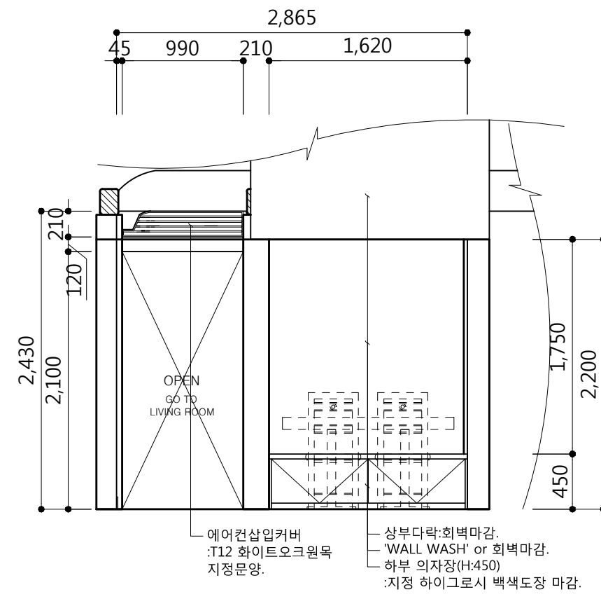
2 | 모던형 주방2안 ELEVATION A
