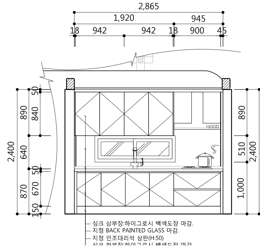
2 모던형 주방1안 ELEVATION A
