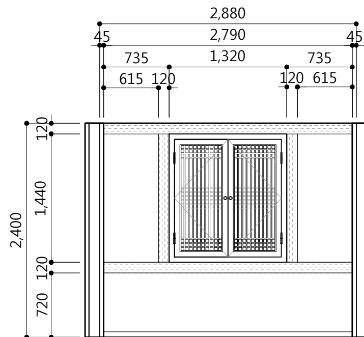
2 전통형 사랑방 ELEVATION A
