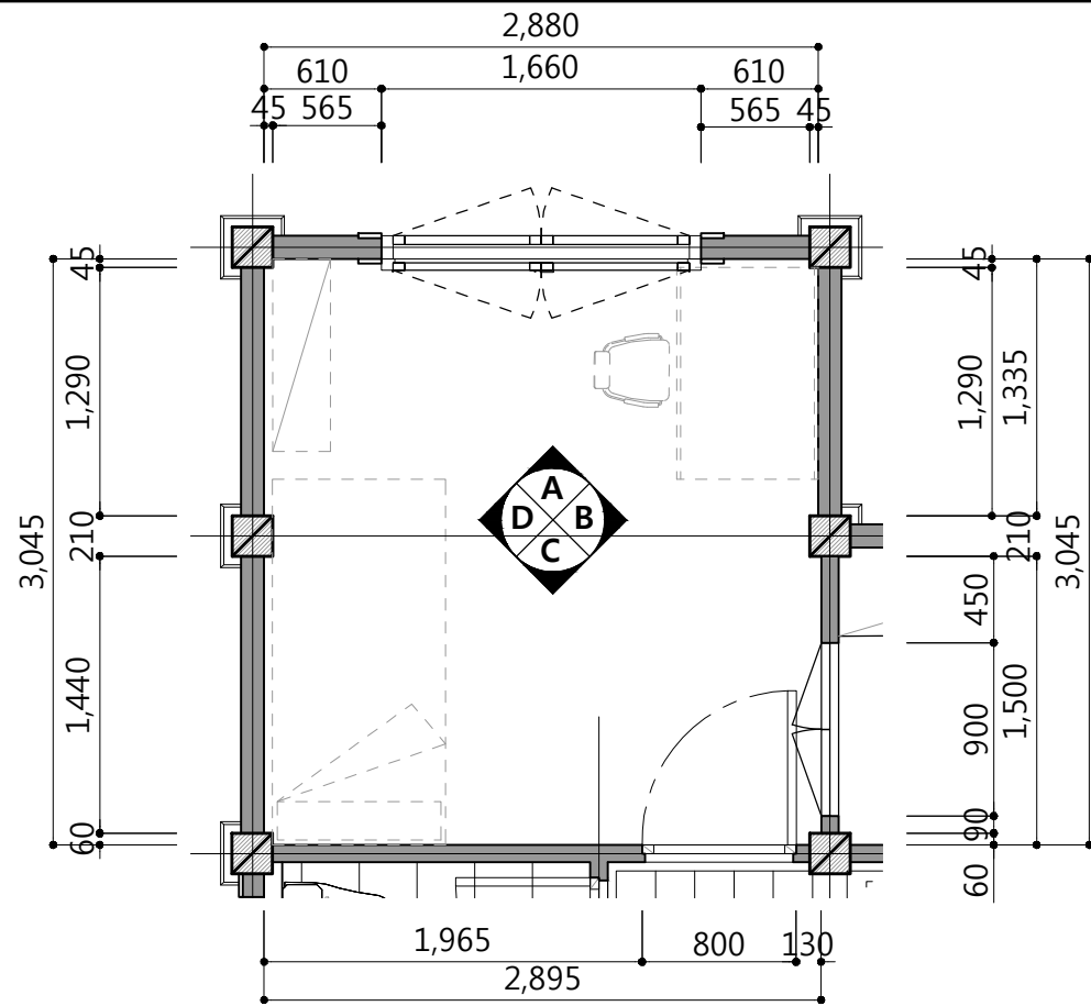
1 전통형 건넌방 TOP PLAN
