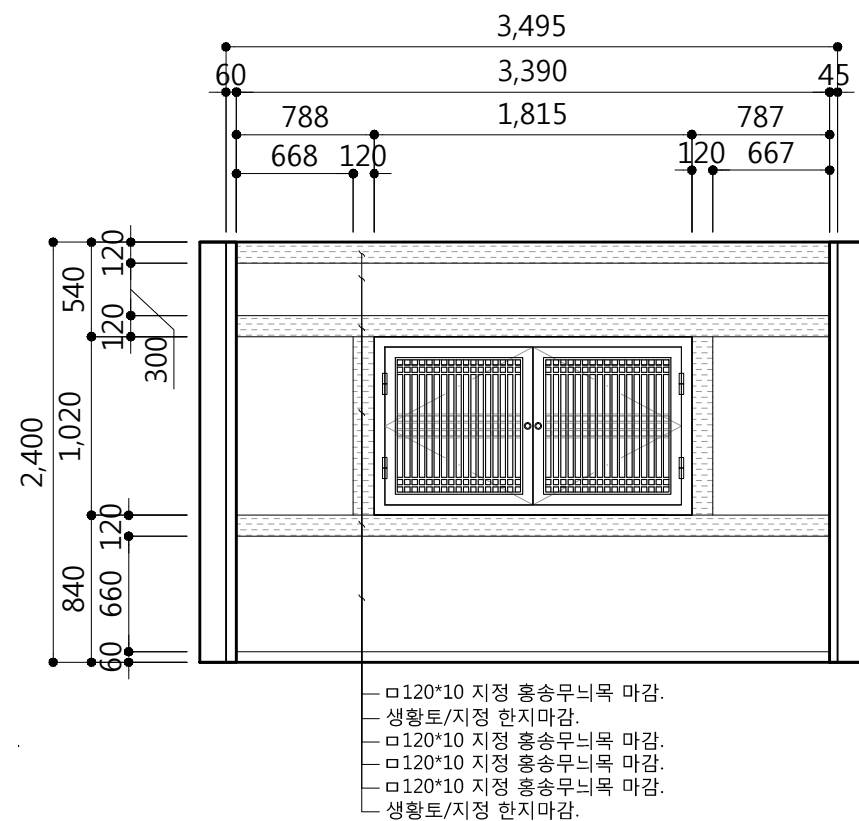
3 전통형 사랑방 ELEVATION B,C,D
