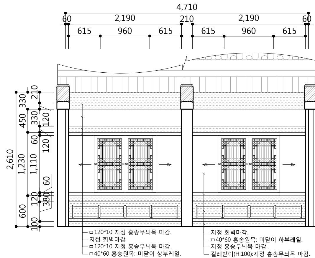
2 전통형 거실 ELEVATION A, A'
