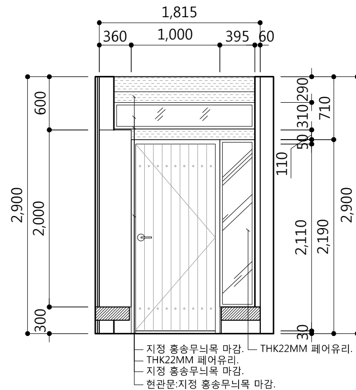
2 전통형 현관 ELEVATION A
