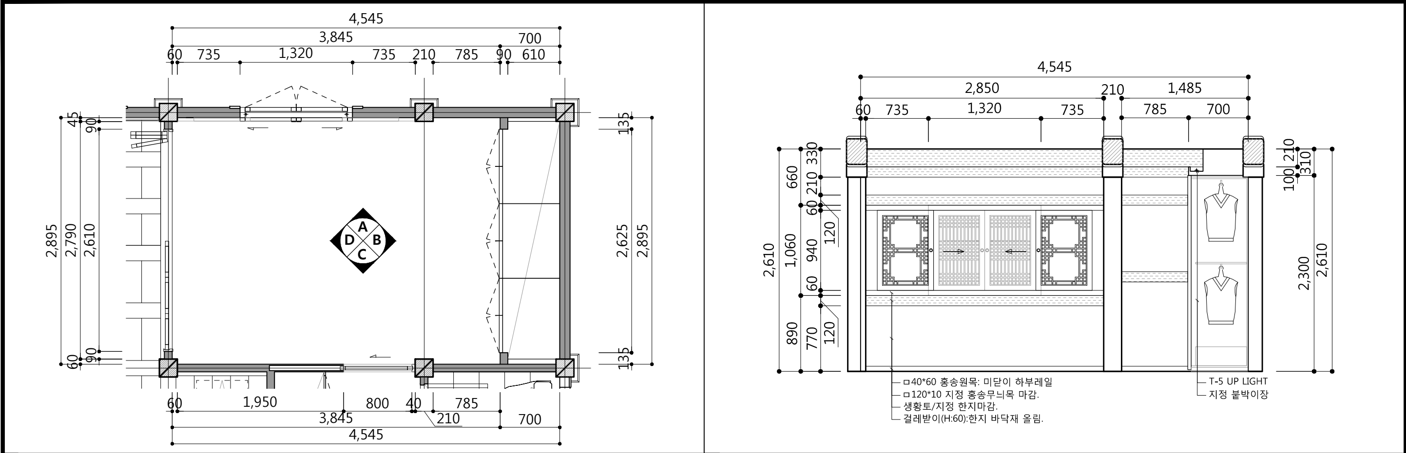
1 전통형 안방 TOP PLAN SCALE-A3:1/40, A4:1/60 2 전통형 안방 ELEVATION A SCALE-A3:1/40, A4:1/60
