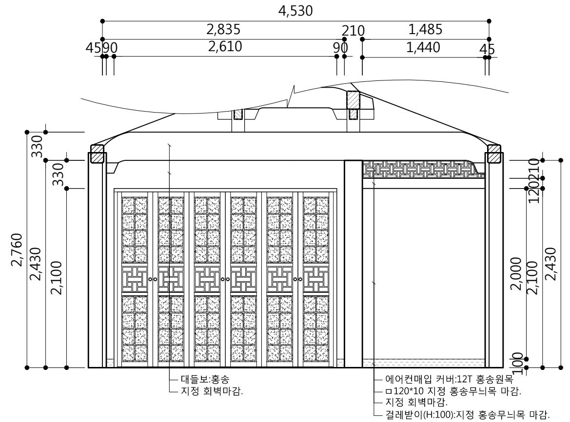
2 전통형 거실 ELEVATION B
