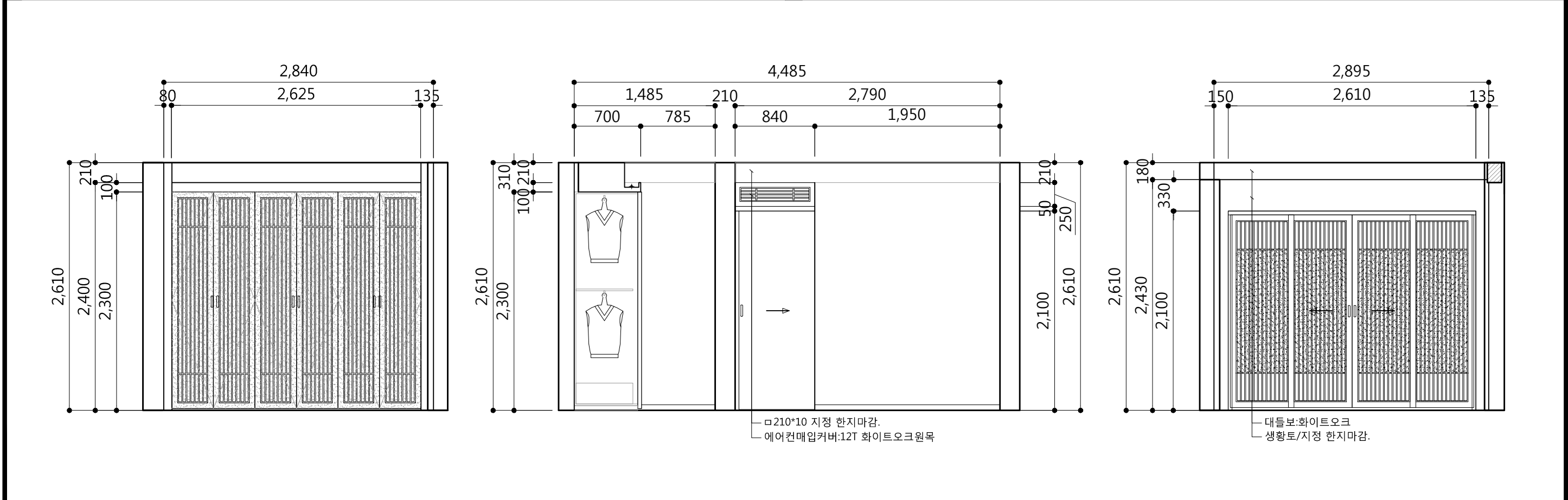
3 모던형 안방 ELEVATION B,C,D SCALE-A3:1/40, A4:1/60
