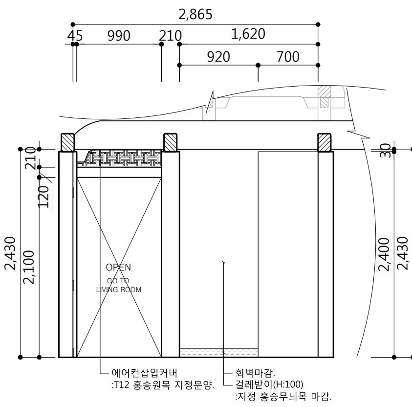
2 전통형 주방1안 ELEVATION A
