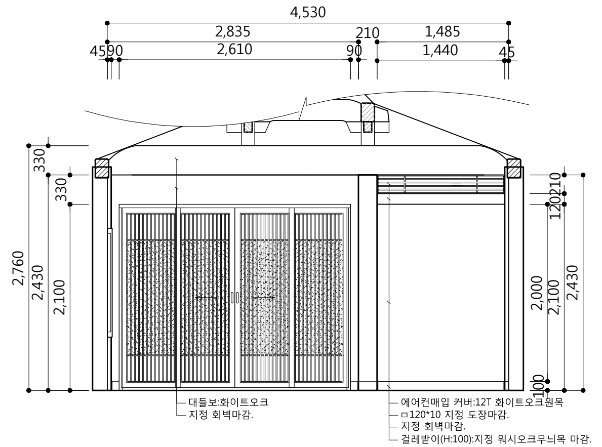
2 | 모던형 거실 ELEVATION B
