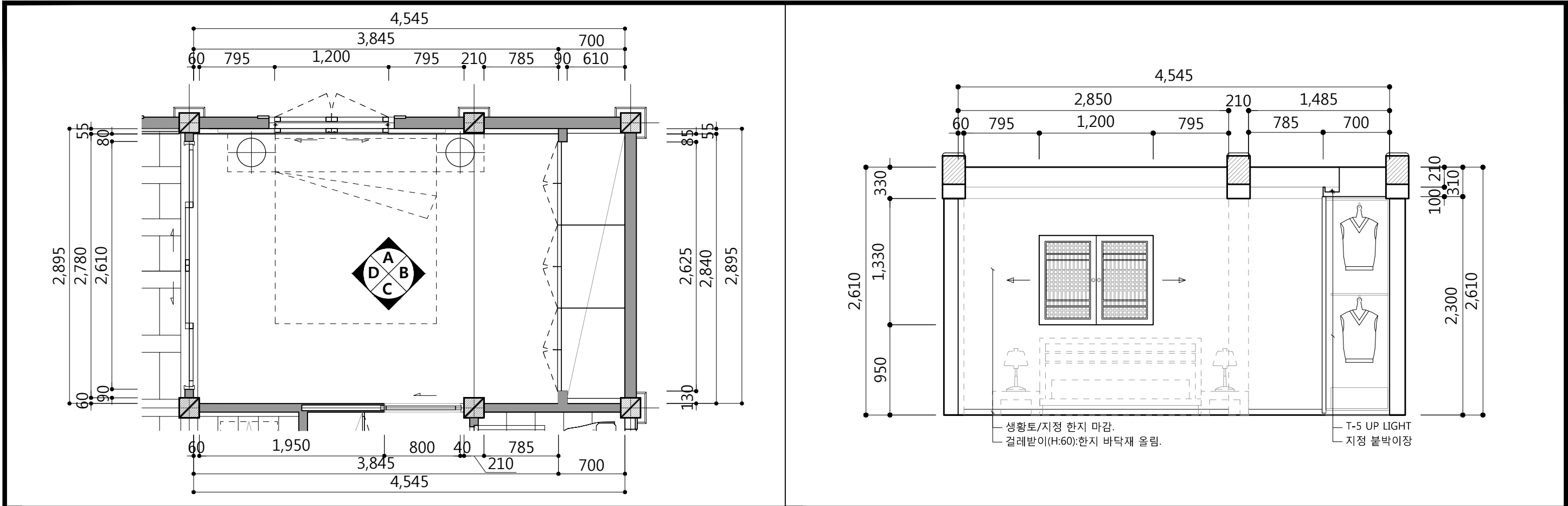
1 모던형 안방 TOP PLAN SCALE-A3:1/40, A4:1/60 2 모던형 안방 ELEVATION A SCALE-A3:1/40, A4:1/60
