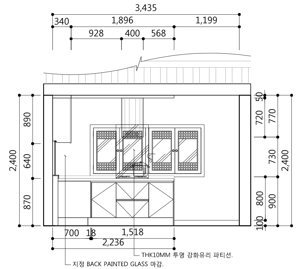
3 | 모던형 주방2안 ELEVATION B,C,D
