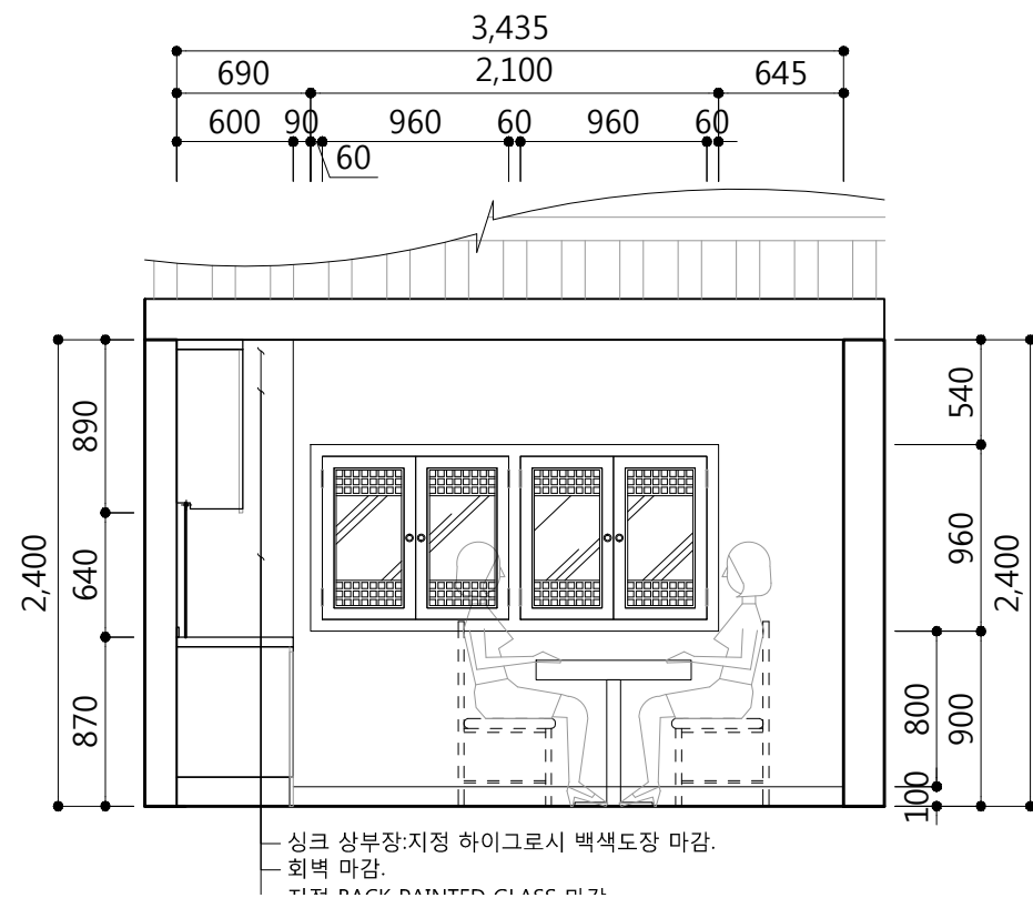
3 모던형 주방1안 ELEVATION B,C,D
