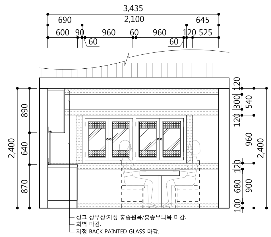
3 전통형 주방1안 ELEVATION B,C,D
