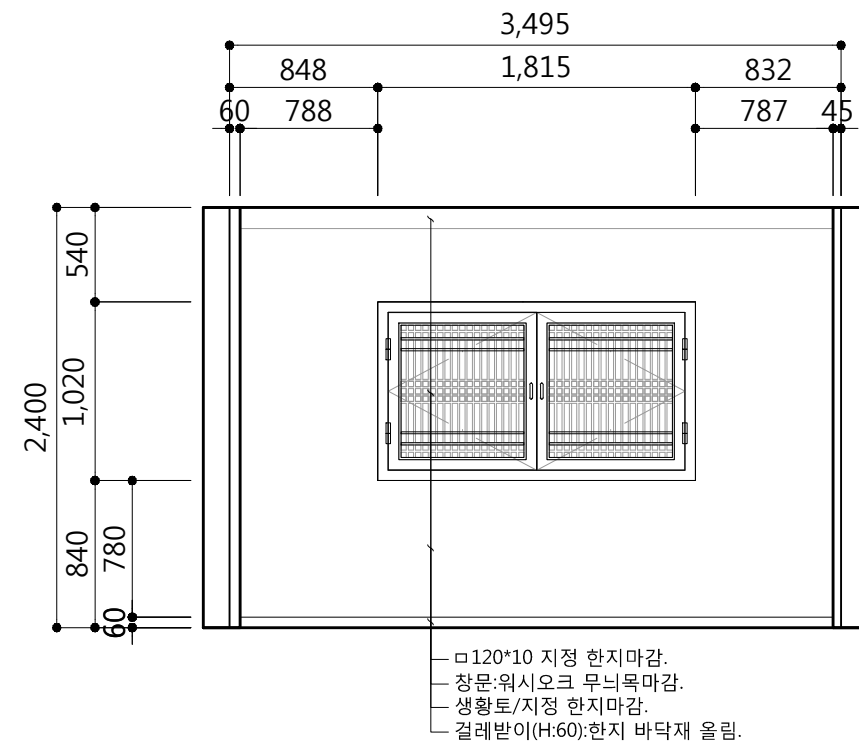
3 모던형 사랑방 ELEVATION B,C,D
