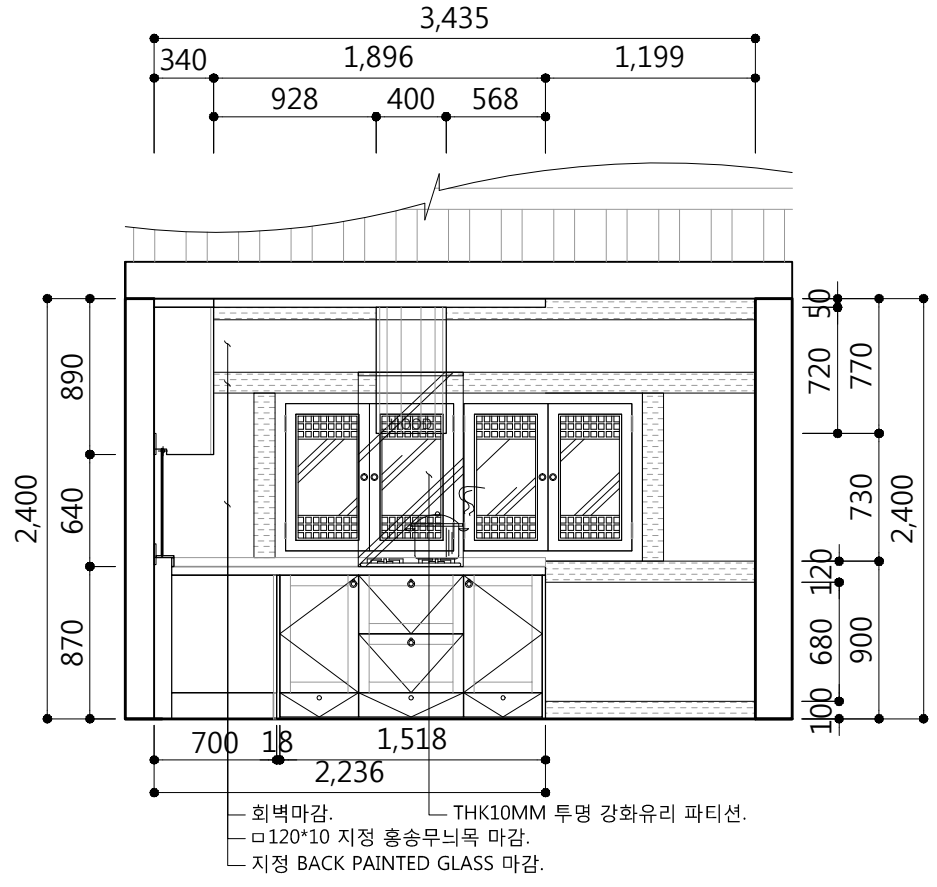
3 전통형 주방2안 ELEVATION B,C,D
