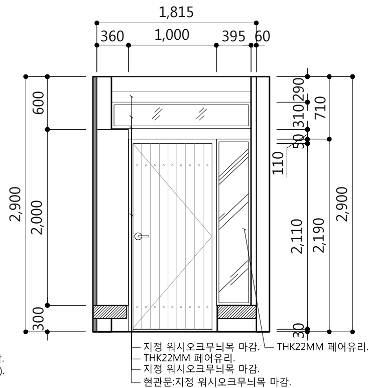
2 모던형 현관 ELEVATION A
